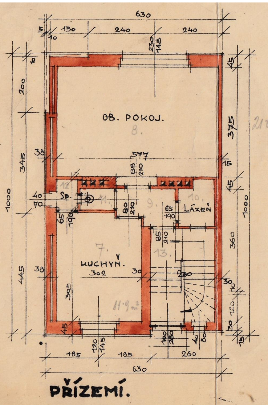
1.NP - STAV
